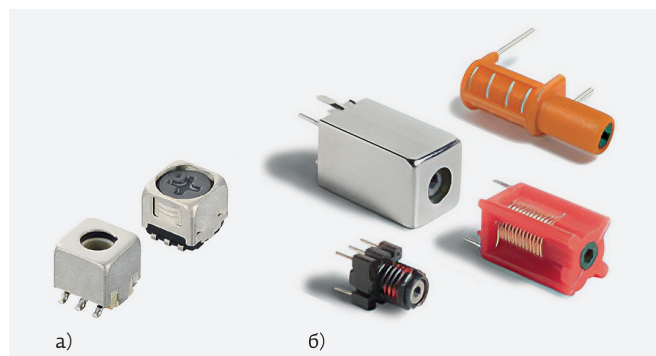
Рис. 28. Сравнение переменных индуктивностей: а – бюджетные переменные индуктивности серий 5CCEG и FSDVA компании Murata; б – подстроечные (tunable) высокочастотные индуктивности серий Uni5, Uni10, Slot7 и 148 компании Coilcraft
