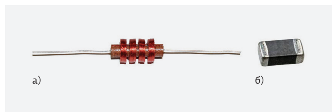
Рис. 27. Внешний вид многослойных дросселей: а – дроссель серии 4021162 «Wilco» компании RF Parts Company; б – многослойный дроссель ТВ1608 компании Murata
