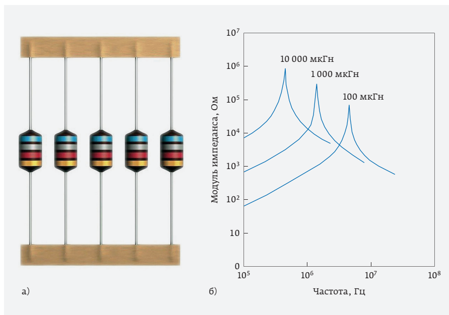
Рис. 24. Дроссель серии HLVC компании TDK: а – внешний вид; б – зависимость модуля импеданса от частоты
